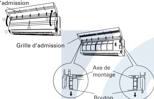
Grille d'admission
