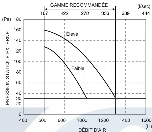
Schéma 50 PERFORMANCE DU VENTILATEUR ET FLUX D'AIR PRESSION STATIQUE EXTERNE (Tension: 230 V)
