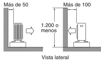
Vista lateral
