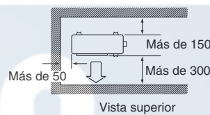
Vista superior
