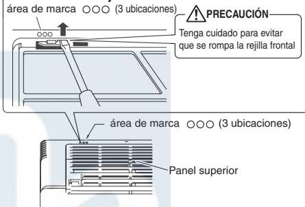
Fig. 2 Ganchos en la rejilla frontal
